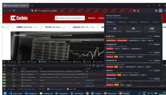
Plugin — aba Terceiros
