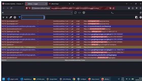
uBlock Origin — logger filtrado (--) com os filtros que bloquearam
