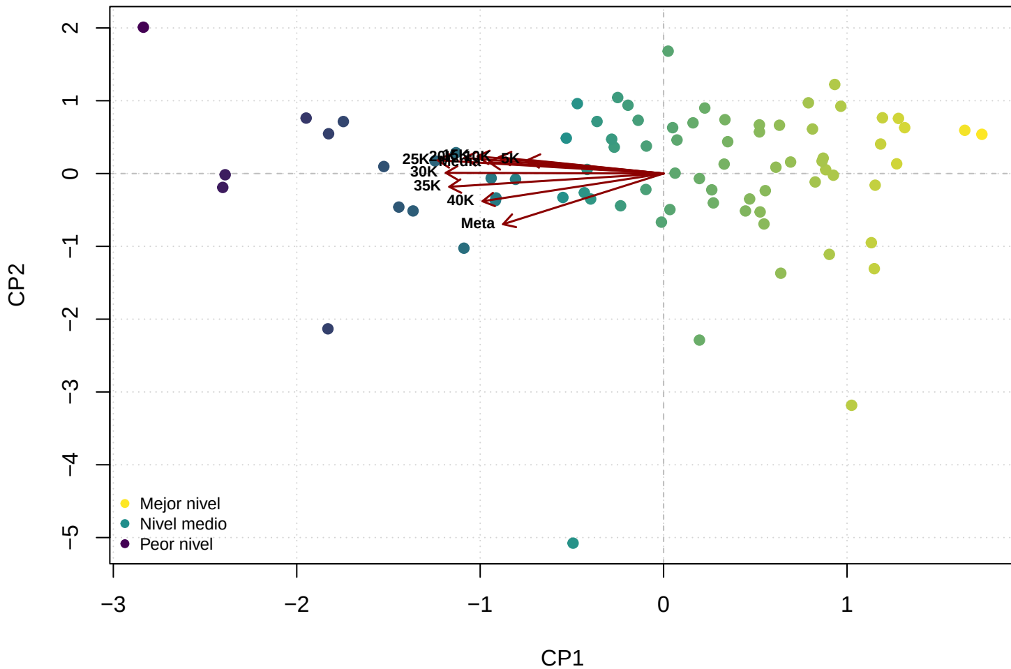
Biplot con gradiente CP1 ( \alpha = 0 )
