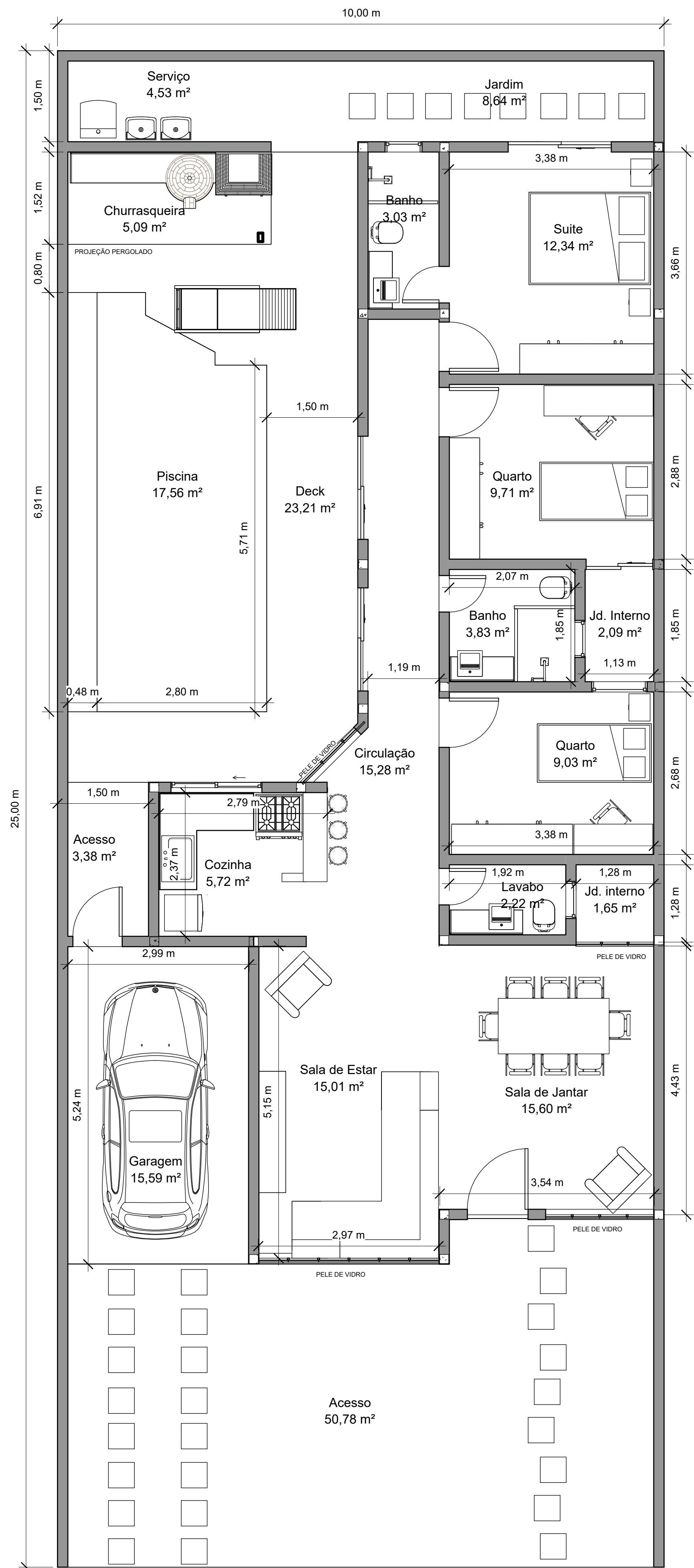
1 TÉRREO PLANTA BAIXA 1 : 50
