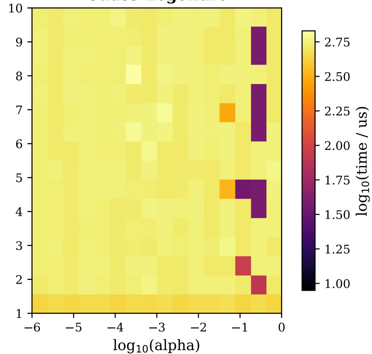
Gauss-Legendre
