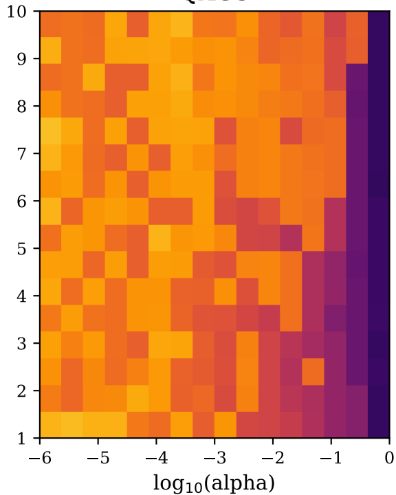
QAGS
