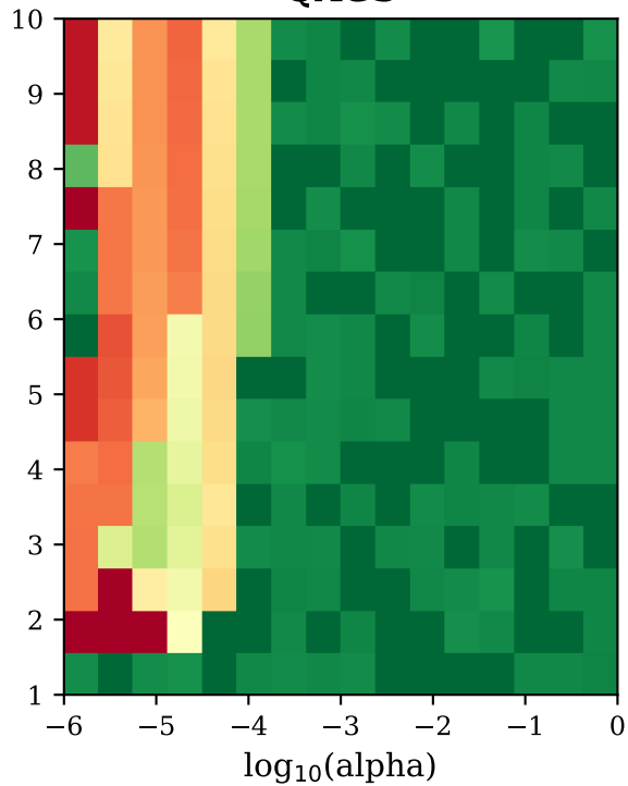
QAGS
