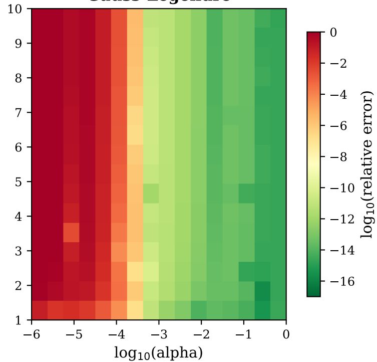
Gauss-Legendre
