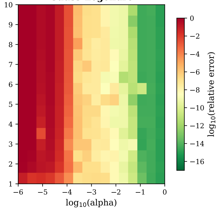
Gauss-Legendre
