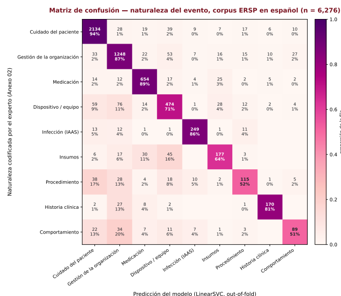
Figura 6. Matriz de confusión de la naturaleza del evento (9 clases) sobre el corpus en español, con predicción fuera de pliegue ( n = 6,276 ). Cada celda muestra el conteo y el porcentaje de la fila; la referencia es la codificación experta (Anexo 02).
