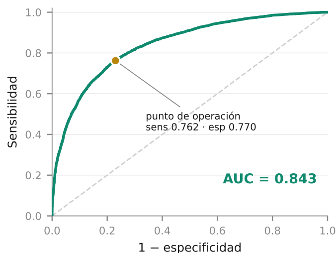
Figura 2. Curva ROC del detector sobre el conjunto de prueba. El punto marcado corresponde al umbral por defecto empleado en operación.
