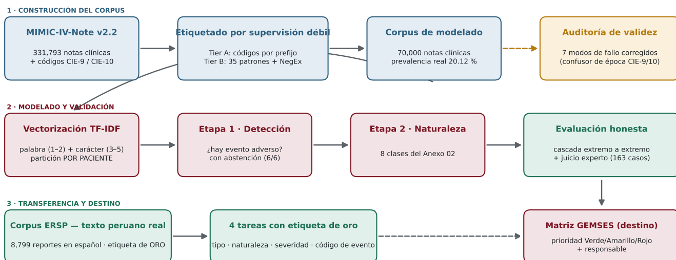
Figura 1. Flujo completo del canal. Banda 1: construcción del corpus por supervisión débil sobre MIMIC-IV-Note, con la auditoría de validez que corrigió siete modos de fallo. Banda 2: modelado en dos etapas con abstención y evaluación honesta (cascada extremo a extremo y contraste con juicio experto). Banda 3: transferencia al español con el corpus ERSP de etiqueta de oro y destino aplicado en la matriz de priorización GEMSES.
