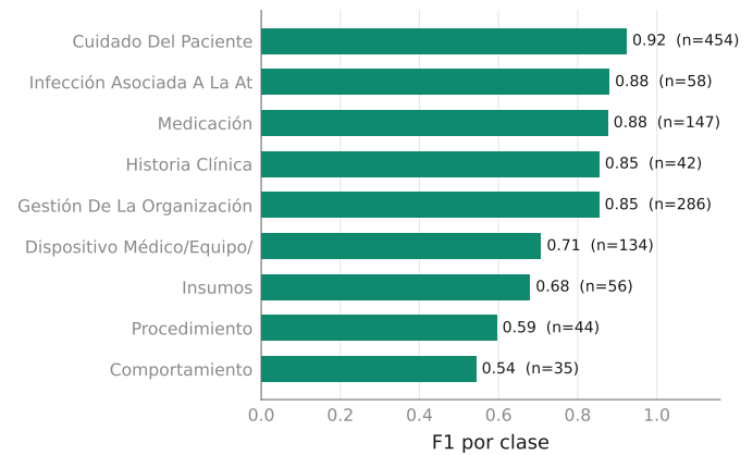
Figura 5. Desempeño por naturaleza del evento sobre el corpus en español con etiqueta de oro. El número de casos de prueba acompaña a cada clase: las de menor F1 son también las de menor soporte.
