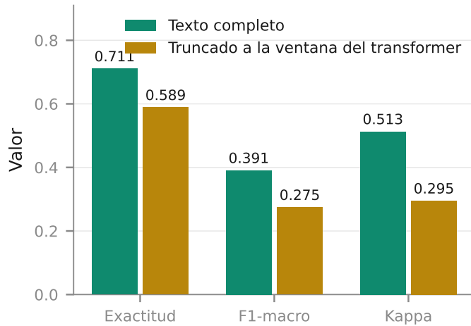
Figura 4. Efecto aislado de la ventana de contexto. Mismo algoritmo y mismos datos; lo único que cambia es cuánto texto procesa el modelo.
