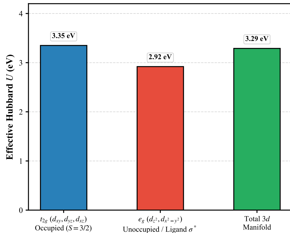
(d) Crystal-Field Orbital Anisotropy in \text{CrCl}_6 Octahedra
