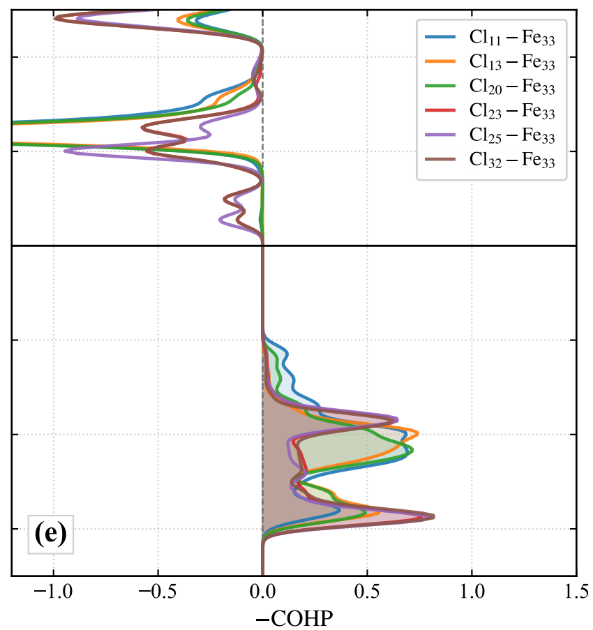
CrCl 3 --Fe (embedded)
