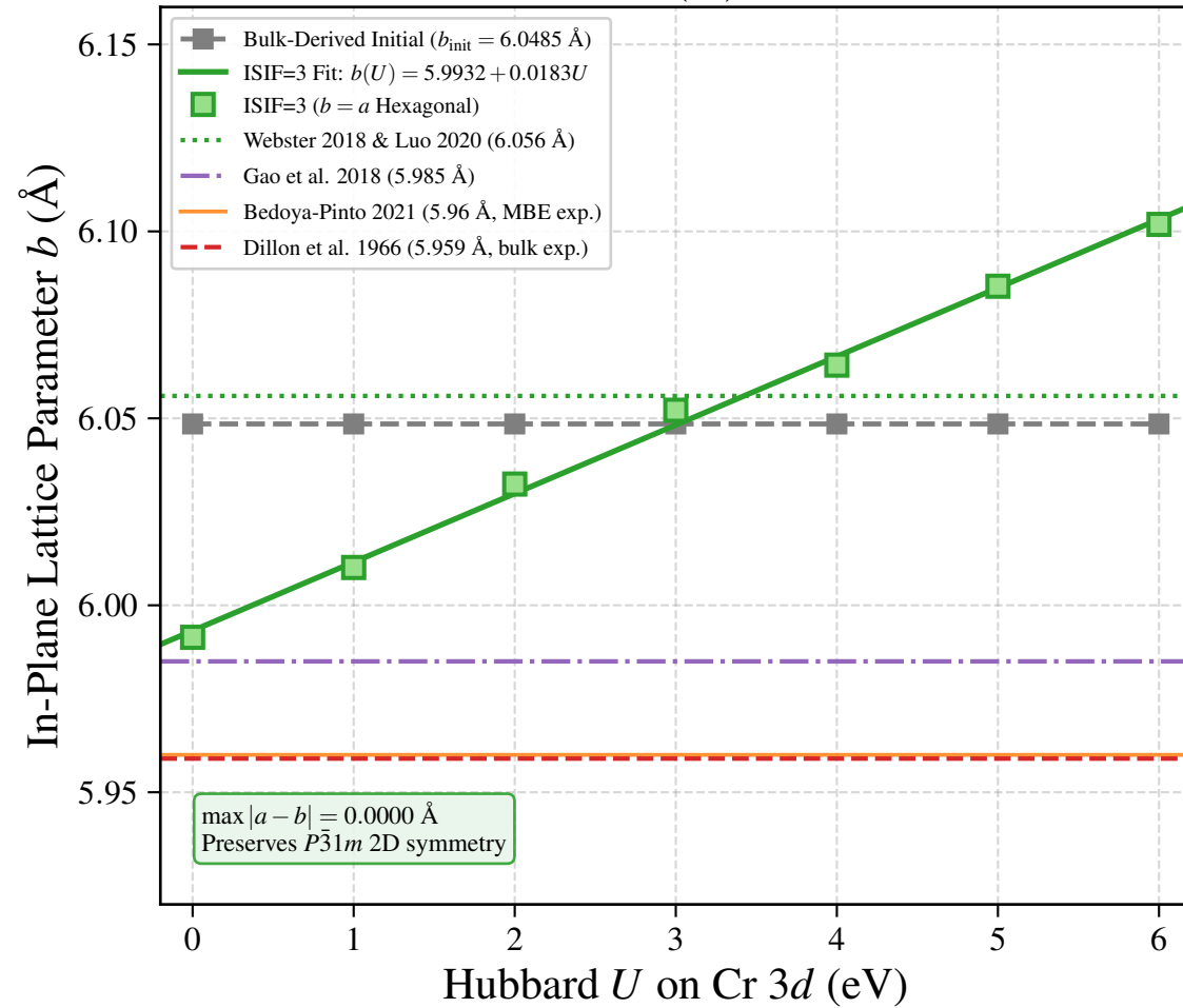
(b) In-Plane Parameter b(U) (Hexagonal Isotropy)
