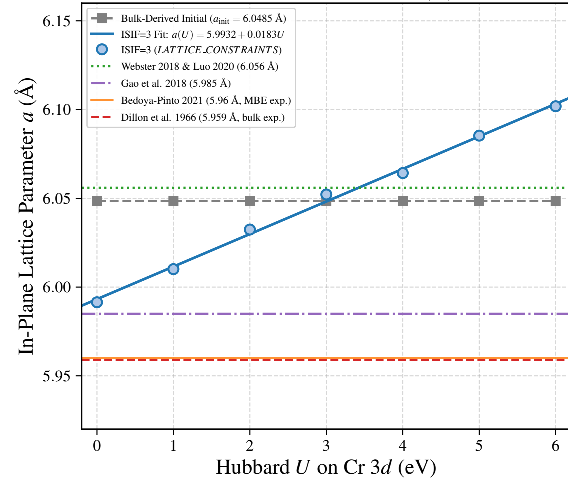
(a) In-Plane Parameter a(U)
