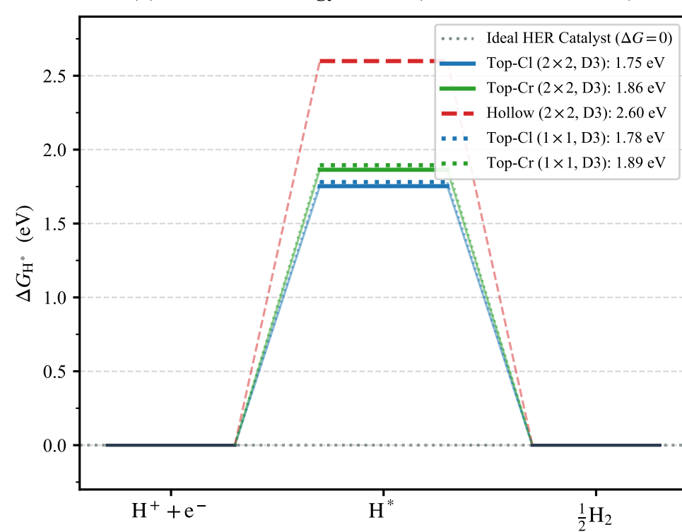
(d) HER Free Energy Profile ( \Delta G_{\text{H}^*} = E_{\text{ads}} + 0.24 eV)
