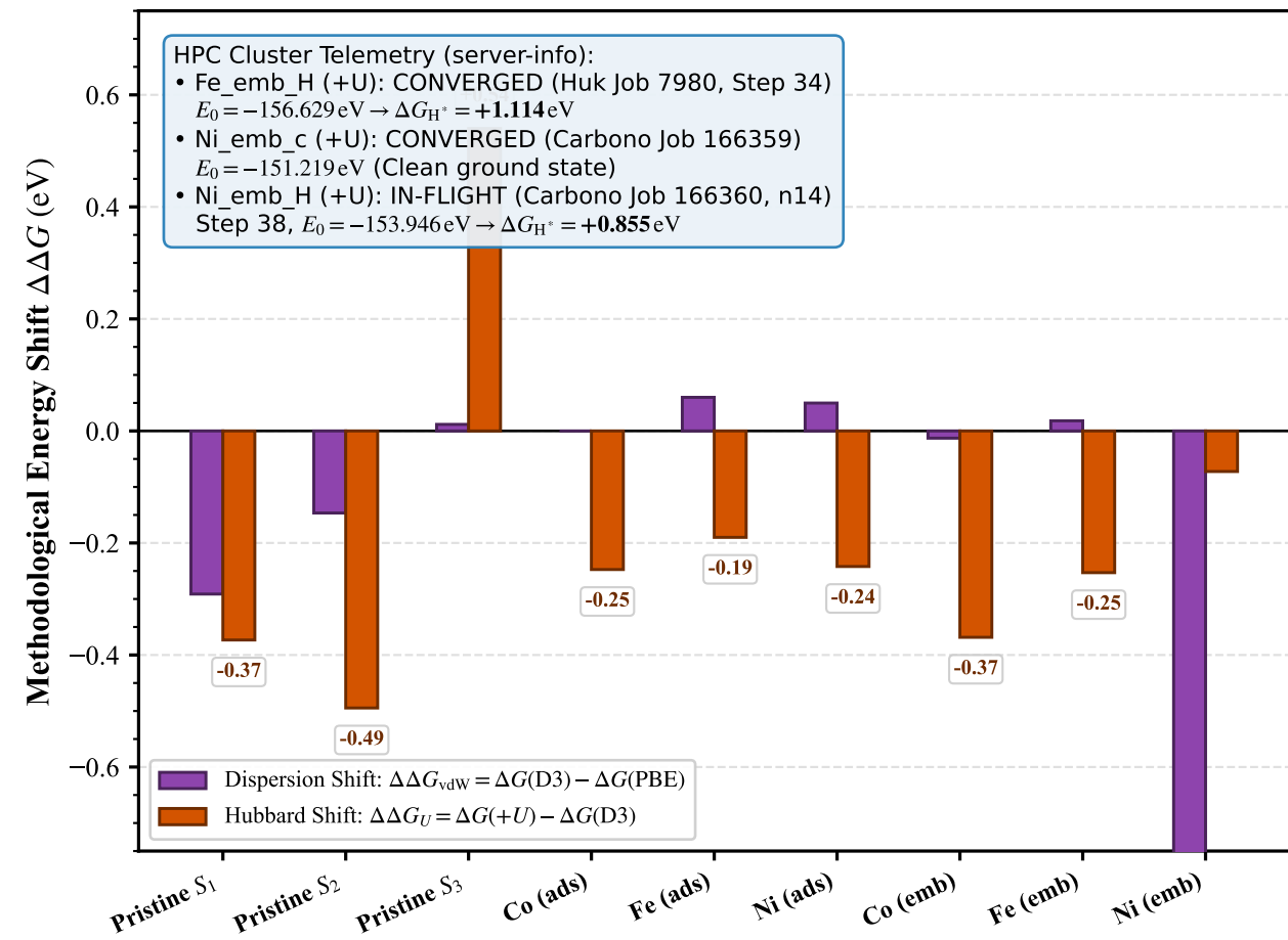
(d) Electronic Stabilization Shifts ( \Delta\Delta G ) & Live HPC Telemetry
