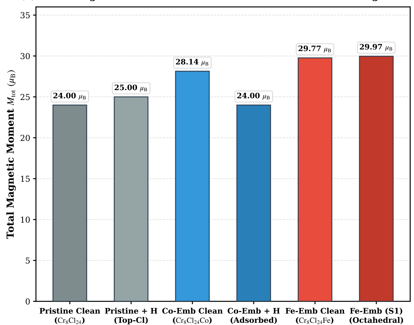
(d) Total Magnetic Moment across Pristine & Embedded Configurations
