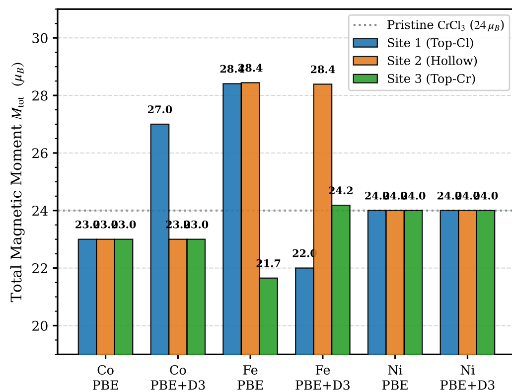
(d) Total Slab Spin Moment M_{\text{tot}} upon TM Adsorption
