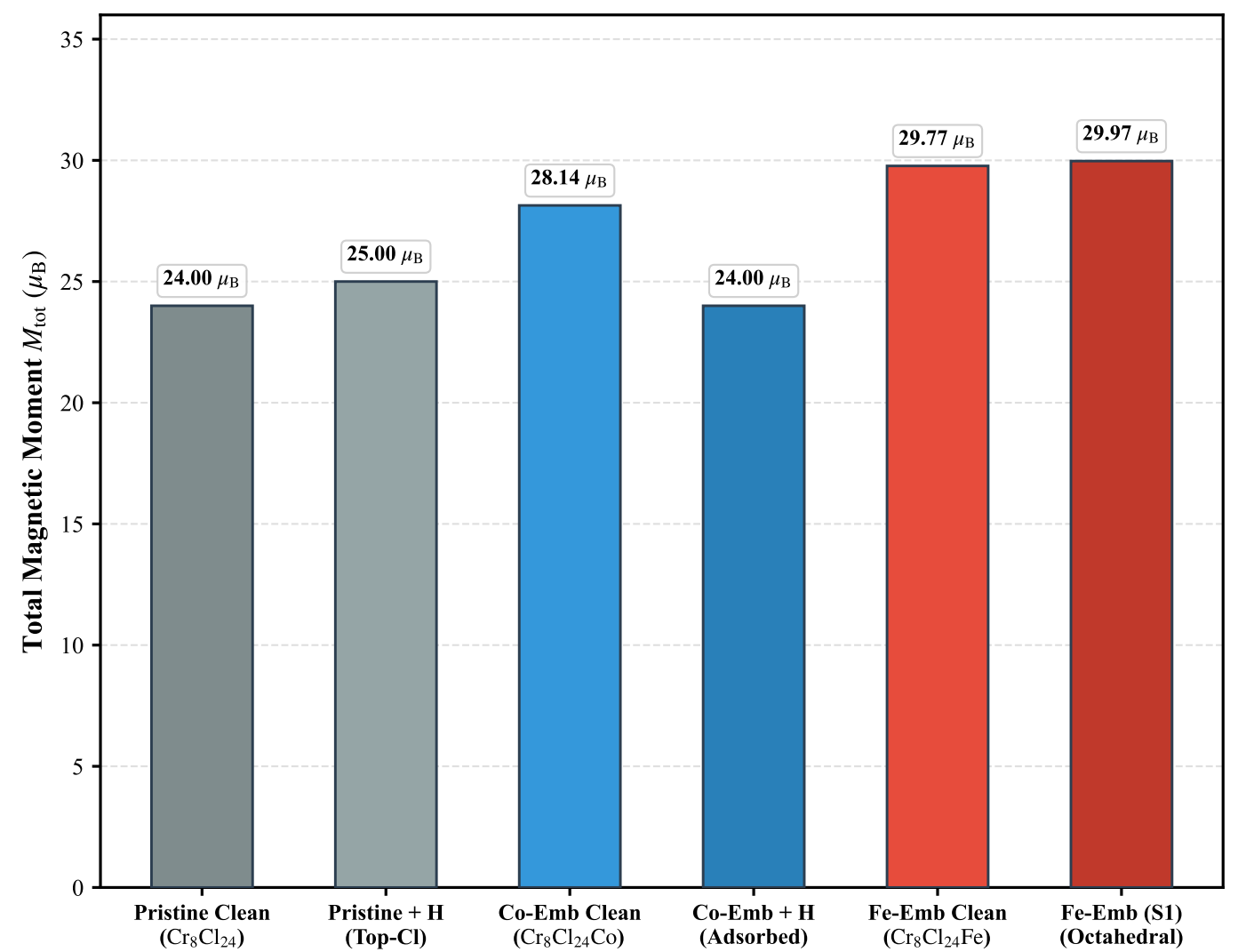
(d) Total Magnetic Moment across Pristine &amp; Embedded Configurations
