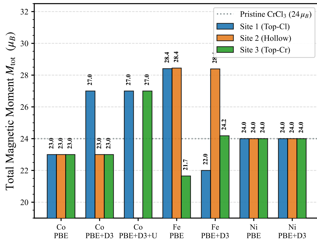
(d) Total Slab Spin Moment M_{\text{tot}} upon TM Adsorption
