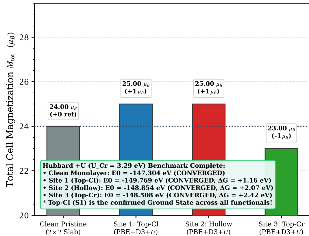
(d) Spin Polarization & Magnetic Compensation ( 2 \times 2 )
