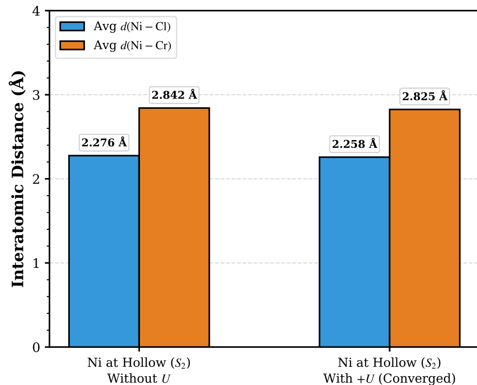
(d) Hollow Coordination Metric under +U
