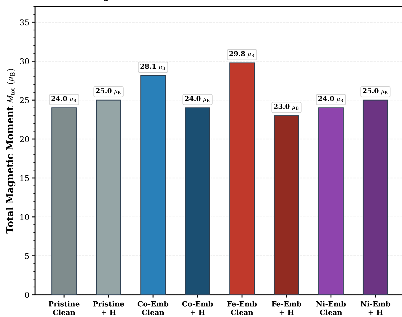
(d) Total Magnetic Moment across Pristine & Embedded Platforms
