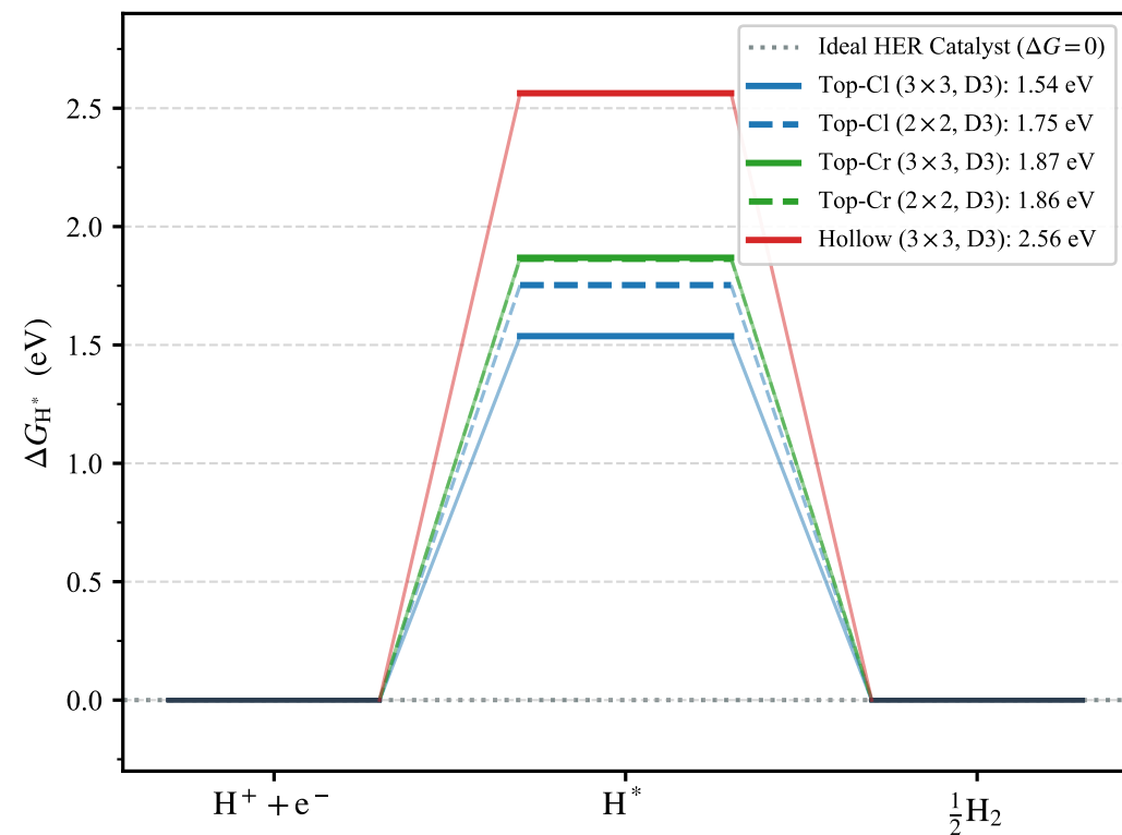
(d) HER Free Energy Profile ( \Delta G_{\text{H}^*} = E_{\text{ads}} + 0.24 eV)
