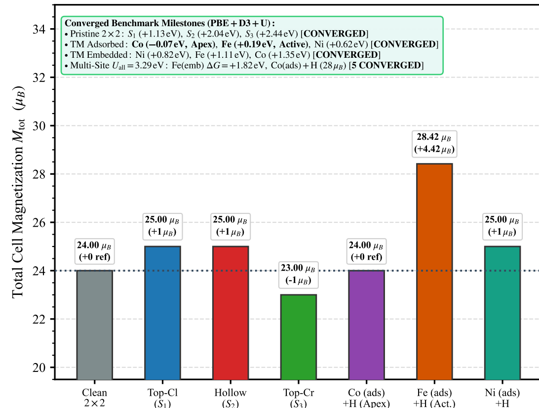
(d) Spin Polarization & Magnetic Compensation ( 2 \times 2 Supercell)
