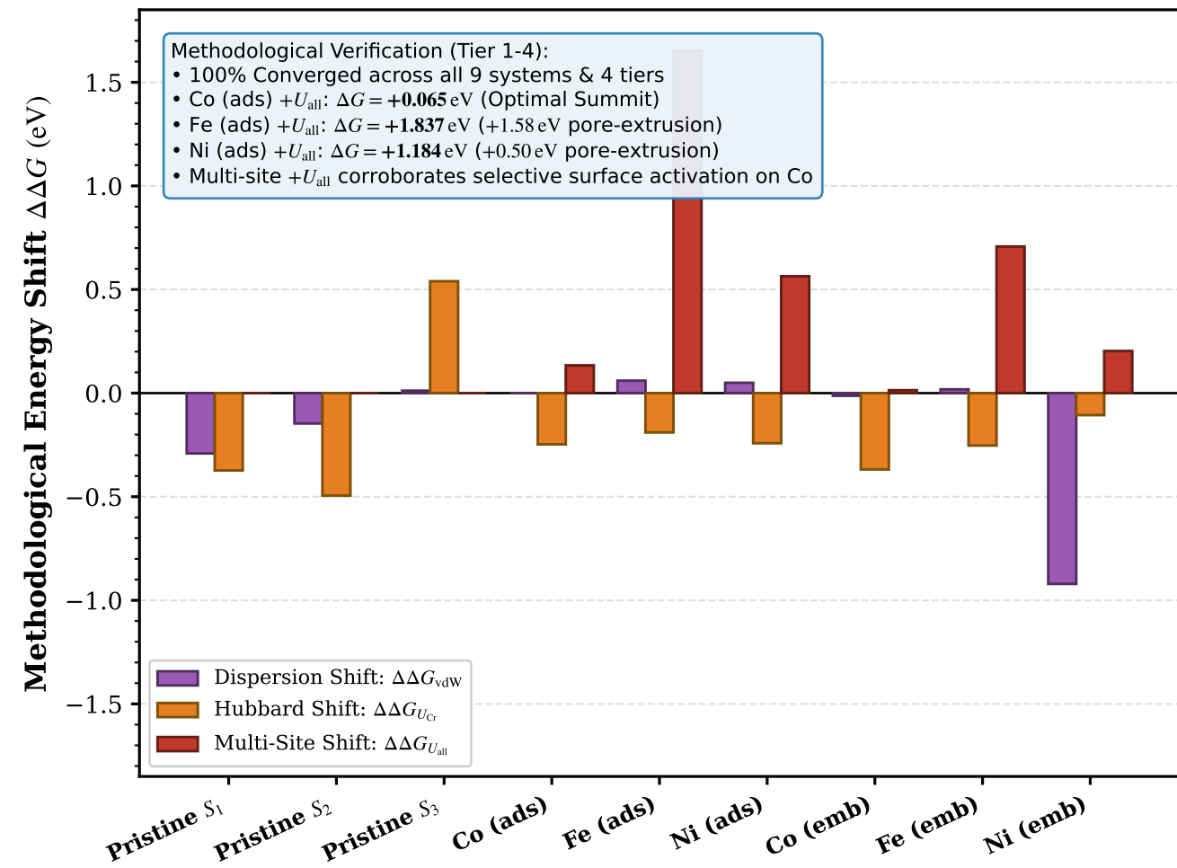
(d) Methodological Energy Shifts ( \Delta\Delta G ) across All Tiers
