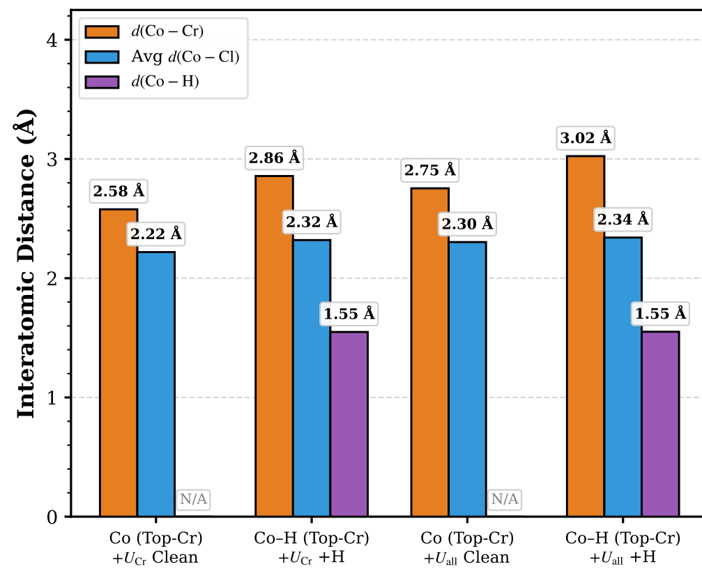
(d) Active Site Coordination Relaxation (+ U_{\text{Cr}} vs + U_{\text{all}} )
