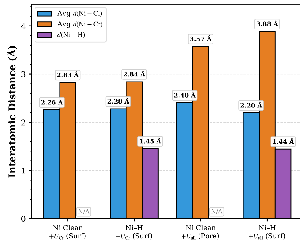
(d) Active Site Geometry: Pore-Sinking vs Surface H Binding
