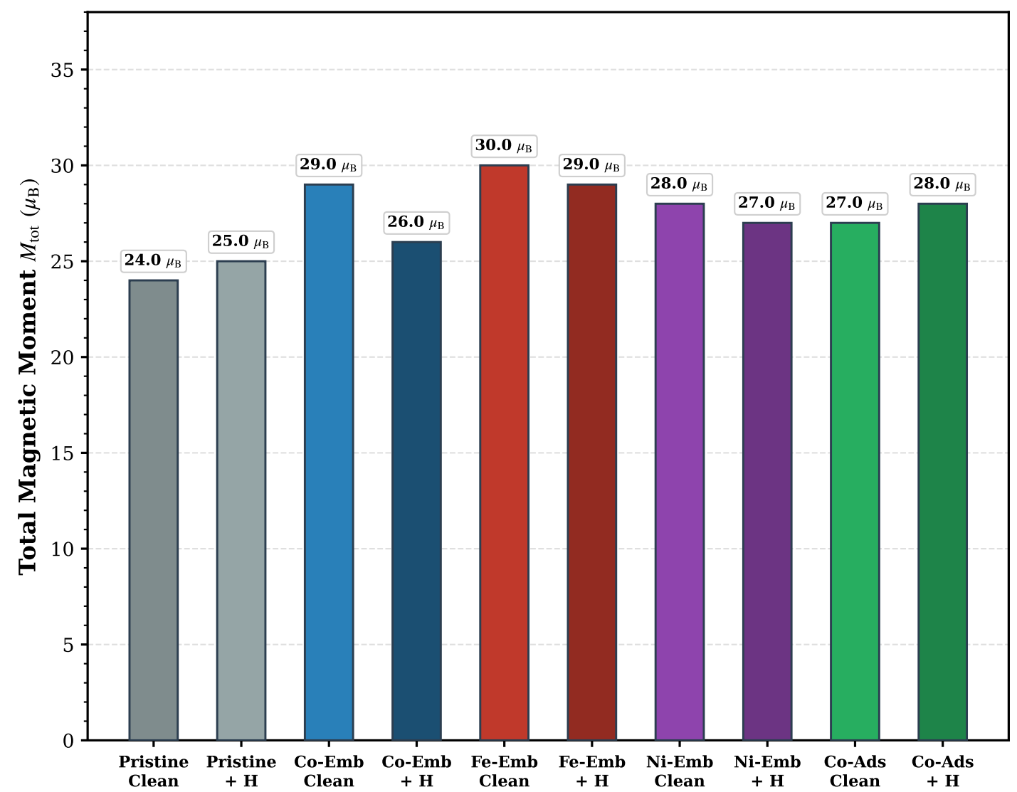
(d) Total Magnetic Moment across Platforms under + U_{\text{all}}
