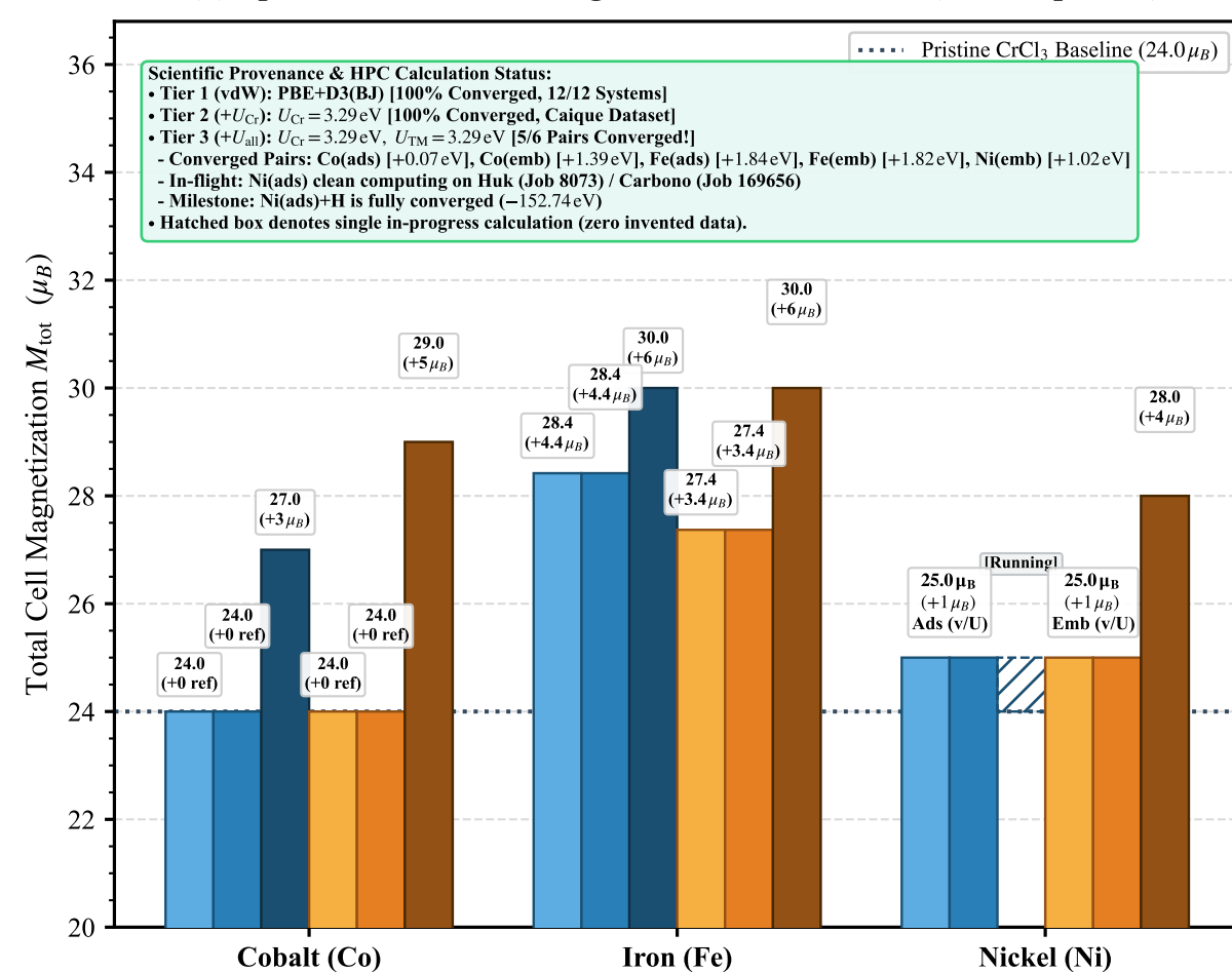
(d) Spin Polarization & Magnetic Moment Trends ( 2 \times 2 Supercell)
