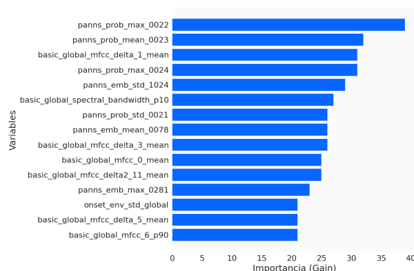
FIGURA 4.14. Top-15 variables predictivas para liveness.
