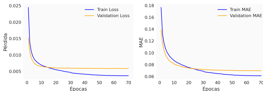
FIGURA 4.1. Curvas de aprendizaje del modelo MLP.
