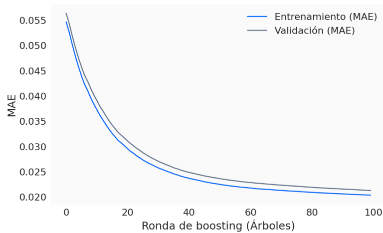
FIGURA 4.4. Curvas de aprendizaje para loudness.
