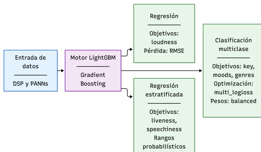
FIGURA 3.13. Resumen del modelado LightGBM.
