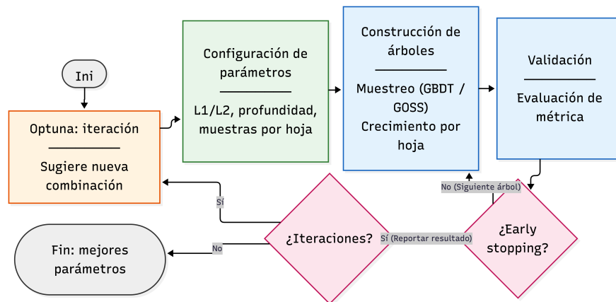
FIGURA 3.14. Flujo de optimización de parámetros para los modelos LightGBM.
