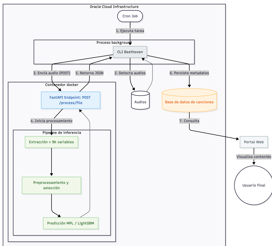
FIGURA 3.12. Arquitectura de despliegue e integración.
