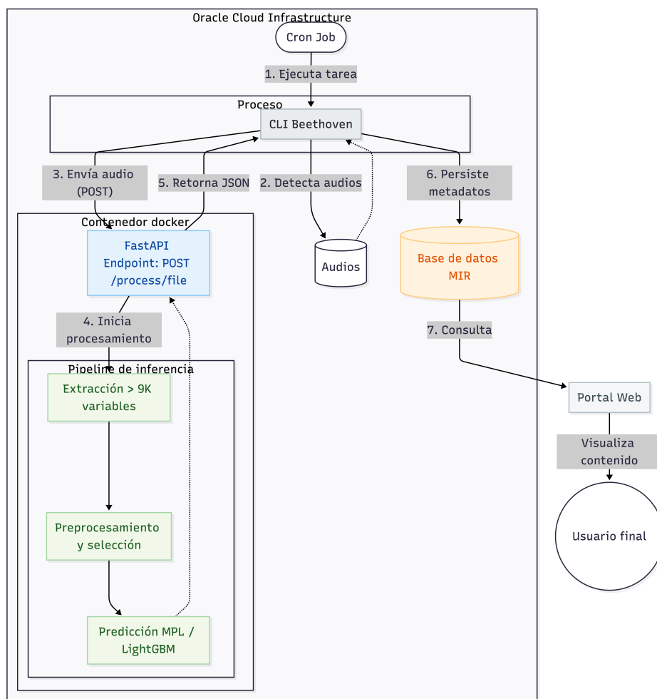
FIGURA 3.15. Diagrama de despliegue e integración.
