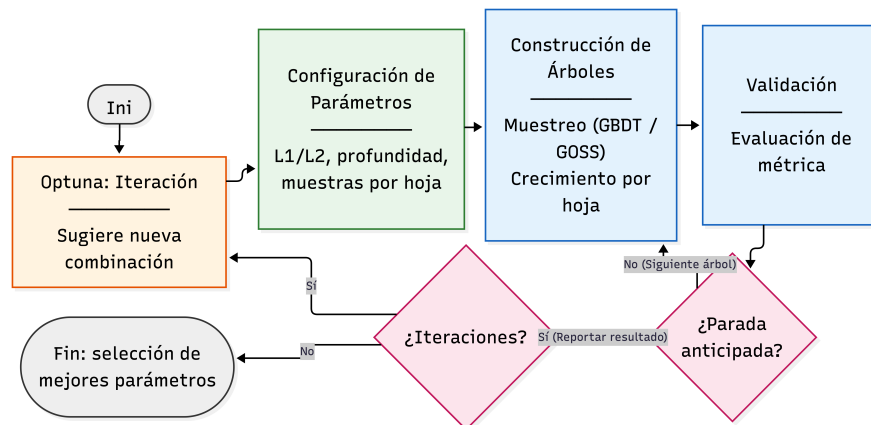
FIGURA 3.14. Resumen del flujo de optimización de parámetros para lightgbm.
