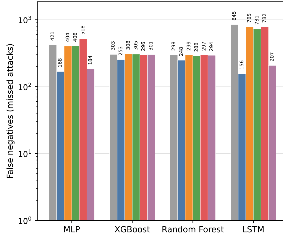
UNSW-NB15
