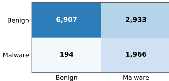
(d) TON_IoT: Best balanced
