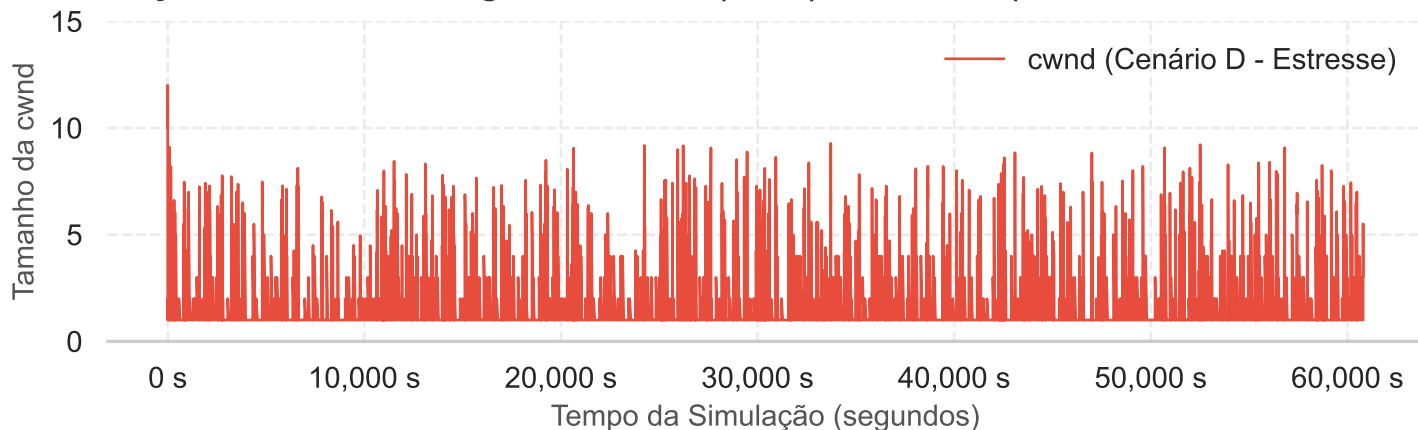
Evolução da Janela de Congestionamento (cwnd) - Cenário D (Perda 20% + Latência 100ms)
