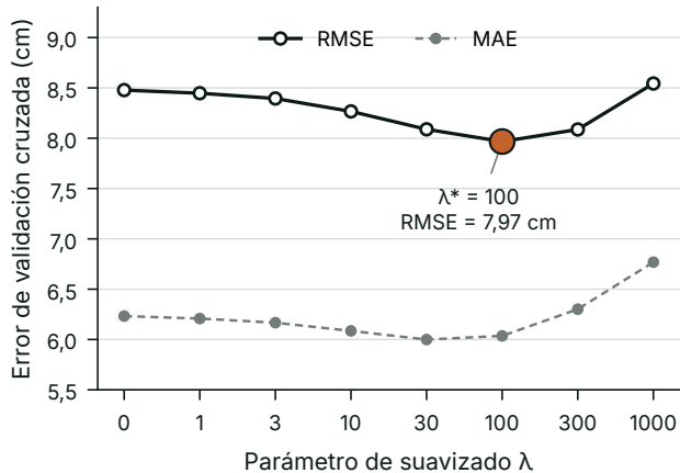
(a) Selección de \lambda por validación cruzada
