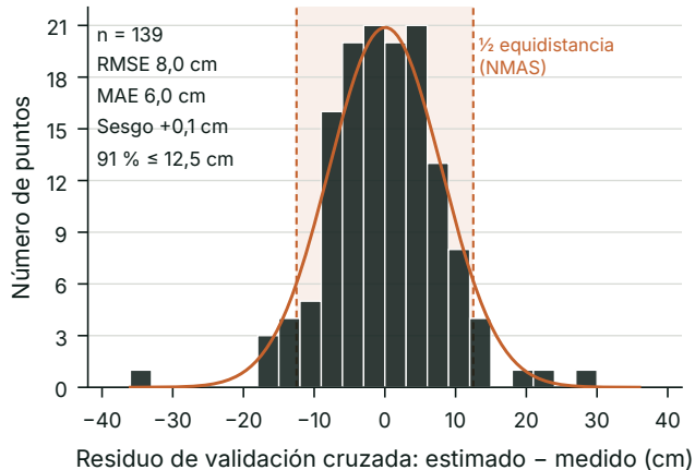
(b) Distribución de los residuos, \lambda = 100
