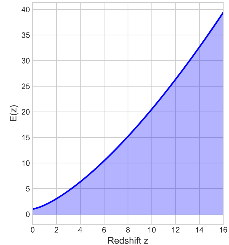
B) Hubble Evolution E(z)
