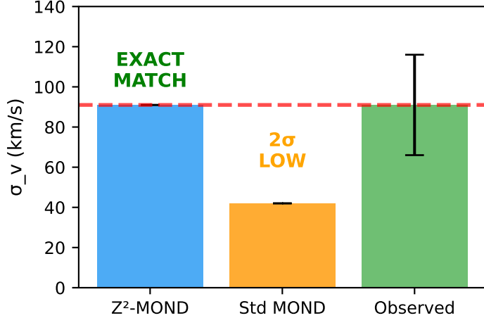
C. GN-z11 (z=10.6)
