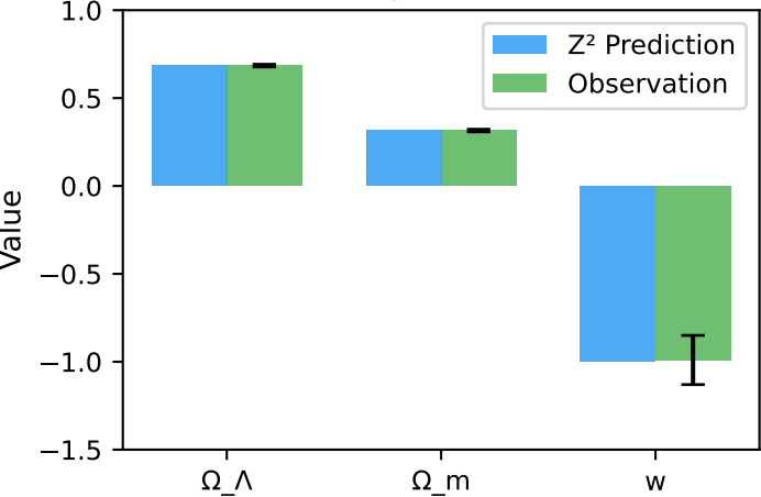
A. Cosmological Parameters
