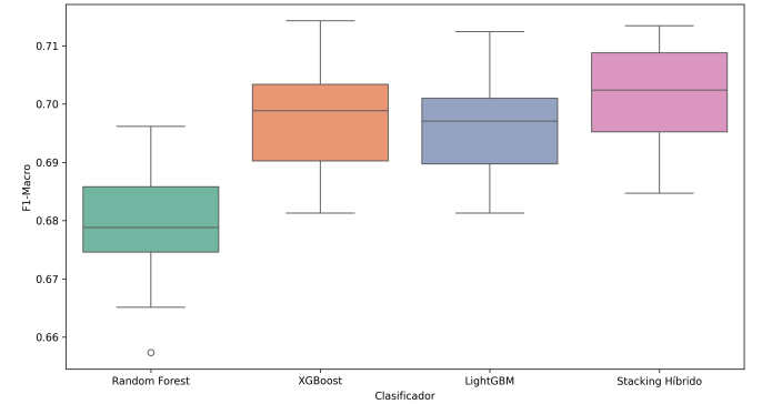
Distribución del F1-Macro en 30 Bloques de Prueba (Validación Estadística)
