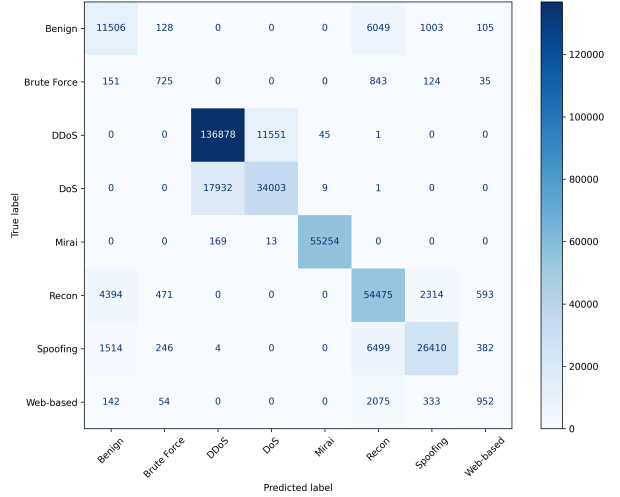
Matriz de Confusión - Stacking Híbrido Propuesto (Meta-LightGBM)
