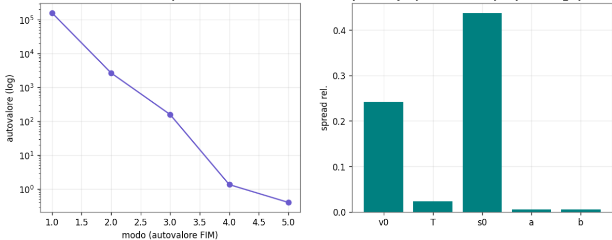
Figura 4.3 - Analisi di identificabilità via FIM: sensibilità per parametro e struttura di correlazione (il mal-condizionamento è la ragione fisica dell'equifinalità).
