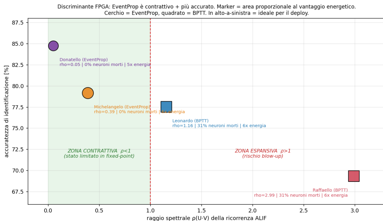
Figura 9.3 - Il discriminante FPGA in un solo grafico: raggio spettrale (x) vs accuratezza (y), area del marker ~ vantaggio energetico. La zona verde ( \rho < 1 ) è quella sicura in fixed-point; Donatello e Michelangelo (cerchi) ci stanno, i BPTT (quadrati) no.
