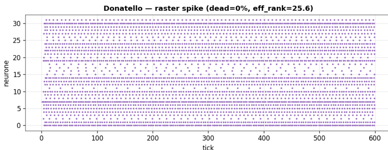
Figura 9.4a - Raster/attività di Donatello (EventProp): attività distribuita su tutti i neuroni, NESSUN neurone spento (0 morti) -- nota: non è iper-sparsa, spara ~19%.
