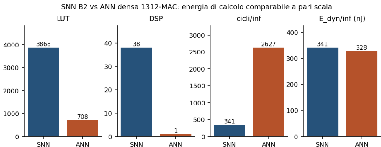
Figura 8.1 — Rete spiking B2 contro rete densa di pari numero di operazioni (1312), stesso flusso di sintesi e stesso clock. L'energia dinamica per inferenza è comparabile (341 contro 328 nJ). Fonte: results.csv, gruppi A e C.
