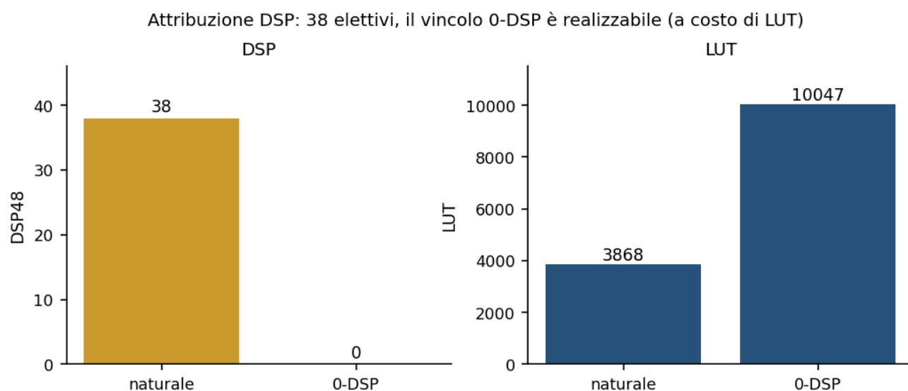
Figura 4.2 — Il compromesso fra blocchi aritmetici e logica: la sintesi naturale usa 38 DSP e 3868 LUT; il vincolo a zero DSP è realizzabile a 10047 LUT. Fonte: results.csv, gruppo A.
