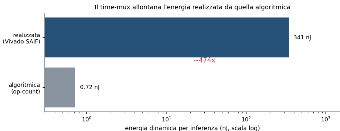
Figura 6.2 — Energia dinamica per inferenza: la realizzazione a moltiplicazione temporale (341 nJ) dista oltre due ordini di grandezza dalla stima algoritmica per conteggio di operazioni (0.72 nJ). Scala logaritmica. Fonte: results.csv, gruppo A.
