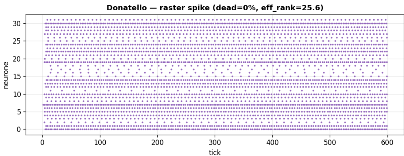
Figura 9.4a - Raster/attivita' di Donatello (EventProp): attivita' distribuita su tutti i neuroni, NESSUN neurone spento (0 morti) -- nota: non e' iper-sparsa, spara \sim 19\% .
