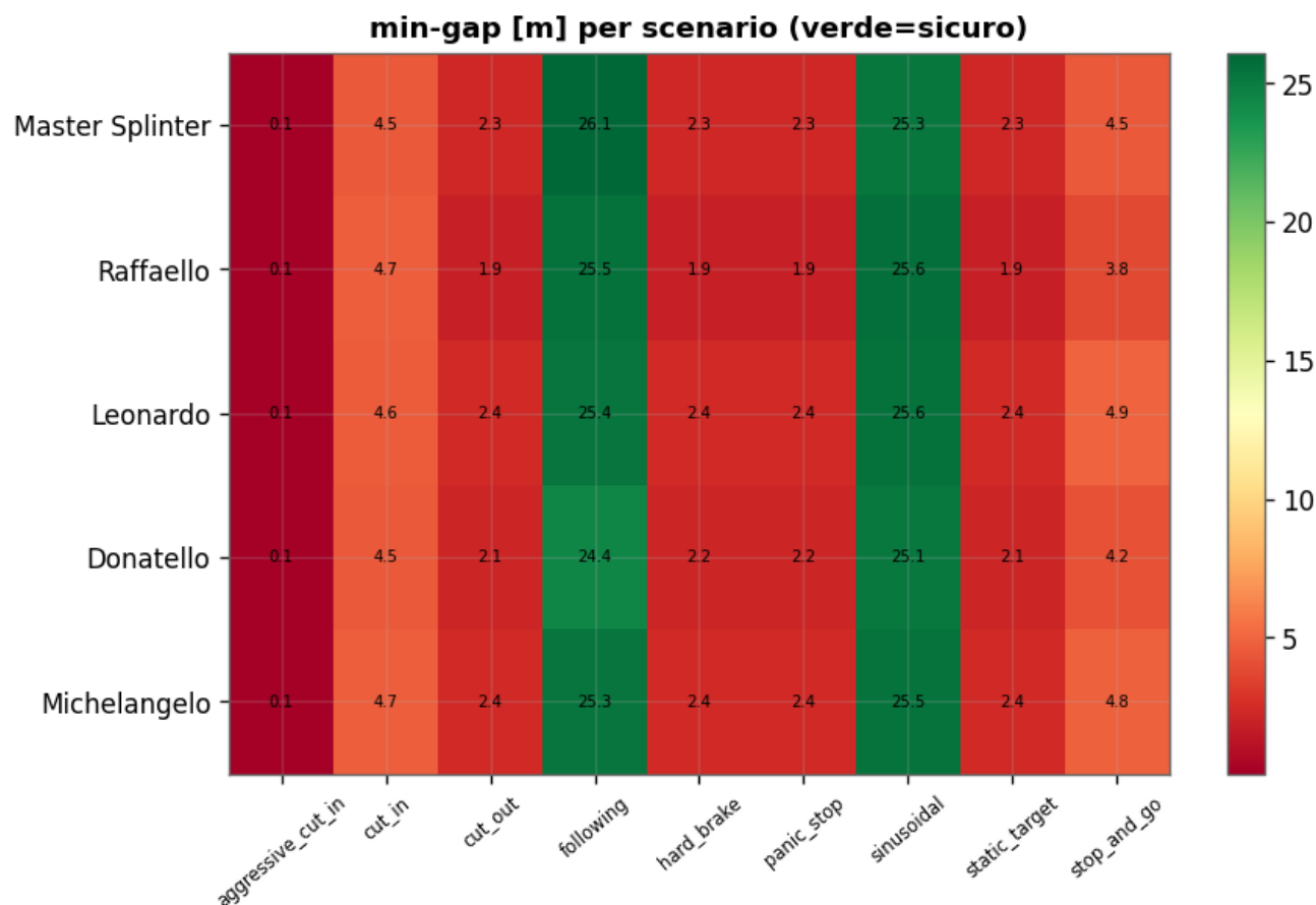
Figura 5.4 - Gap minimo per tipologia di scenario: il cut-in e' il piu' stressante, ma il gap resta sopra la linea di collisione tranne nelle geometrie impossibili.
