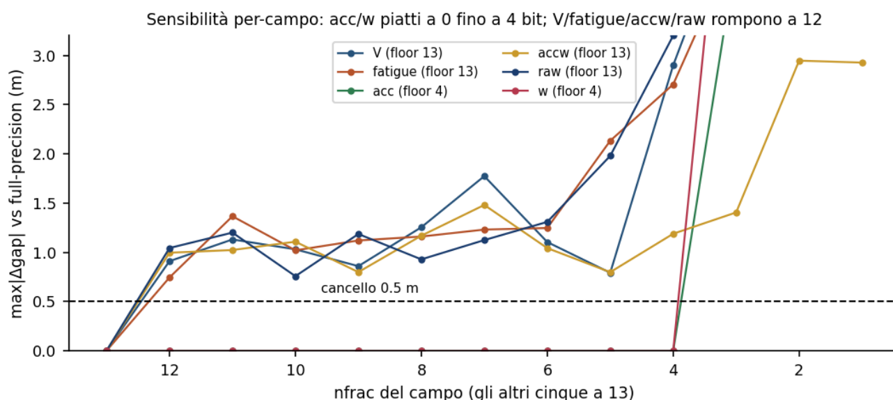
Figura 8.1 — Sensibilità per-campo: scarto massimo del gap quando si abbassa il nfrac di un solo campo, tenendo gli altri cinque a tredici. acc e w restano a zero (bit-identici) fino a quattro bit, poi saltano; V, fatigue, accw e raw superano il cancello già al primo bit tolto. Fonte: mp_sens.tsv.
