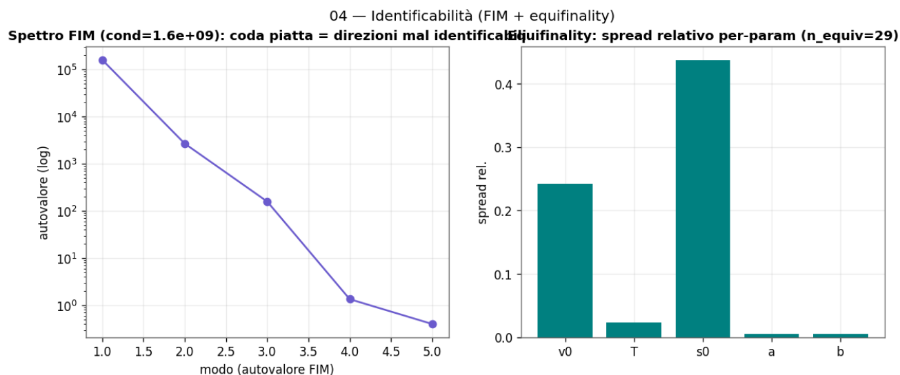
Figura 4.3 - Analisi di identificabilità via FIM: sensibilità per parametro e struttura di correlazione (il mal-condizionamento e' la ragione fisica dell'equifinalità).
