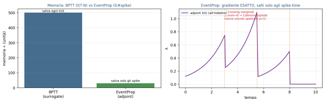
Figura 8.1 — EventProp. A sinistra: memoria O(\#\text{spike}) contro O(T \cdot N) del BPTT. A destra: la variabile aggiunta \lambda è propagata all'indietro e "salta" solo agli istanti di spike.
