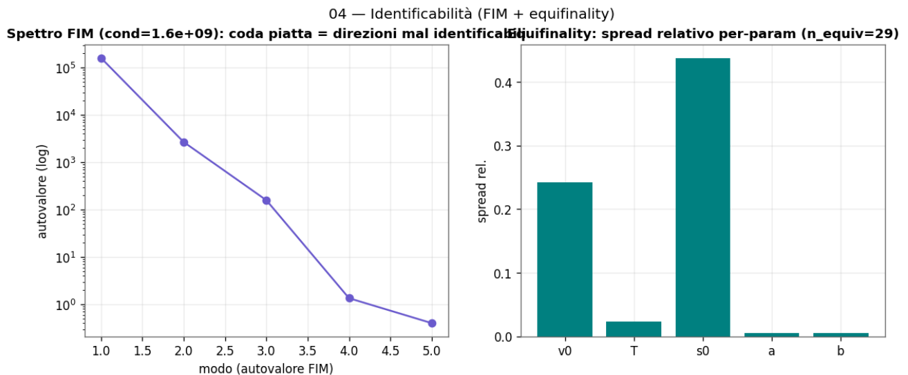
Figura 4.3 - Analisi di identificabilità via FIM: sensibilità per parametro e struttura di correlazione (il mal-condizionamento e' la ragione fisica dell'equifinalità').
