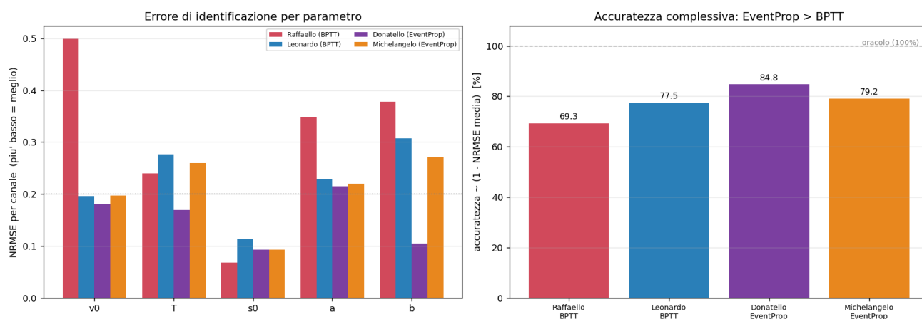
Figura 4.1 - Errore per parametro (sx) e accuratezza complessiva (dx). I due champion EventProp (Donatello viola, Michelangelo arancione) hanno NRMSE per-canale piu' uniforme e bassa; Raffaello (rosso) crolla su v0. La linea tratteggiata a 100% e' l'oracolo.
