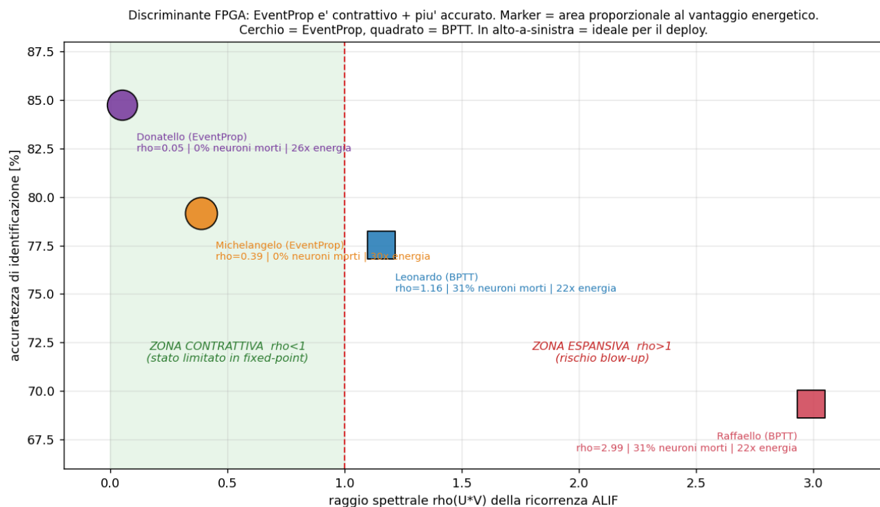
Figura 9.3 - Il discriminante FPGA in un solo grafico: raggio spettrale (x) vs accuratezza (y), area del marker \sim vantaggio energetico. La zona verde ( \rho < 1 ) e' quella sicura in fixed-point; Donatello e Michelangelo (cerchi) ci stanno, i BPTT (quadrati) no.
