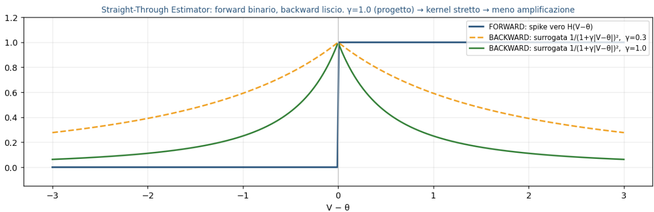
Figura 7.1 — Il meccanismo del surrogate gradient: il forward resta un gradino binario, il backward usa una campana liscia. Con \gamma = 1.0 (verde) il kernel è più stretto che con \gamma = 0.3 , quindi meno neuroni vicini alla soglia contribuiscono al gradiente, con minor rischio di esplosione.
