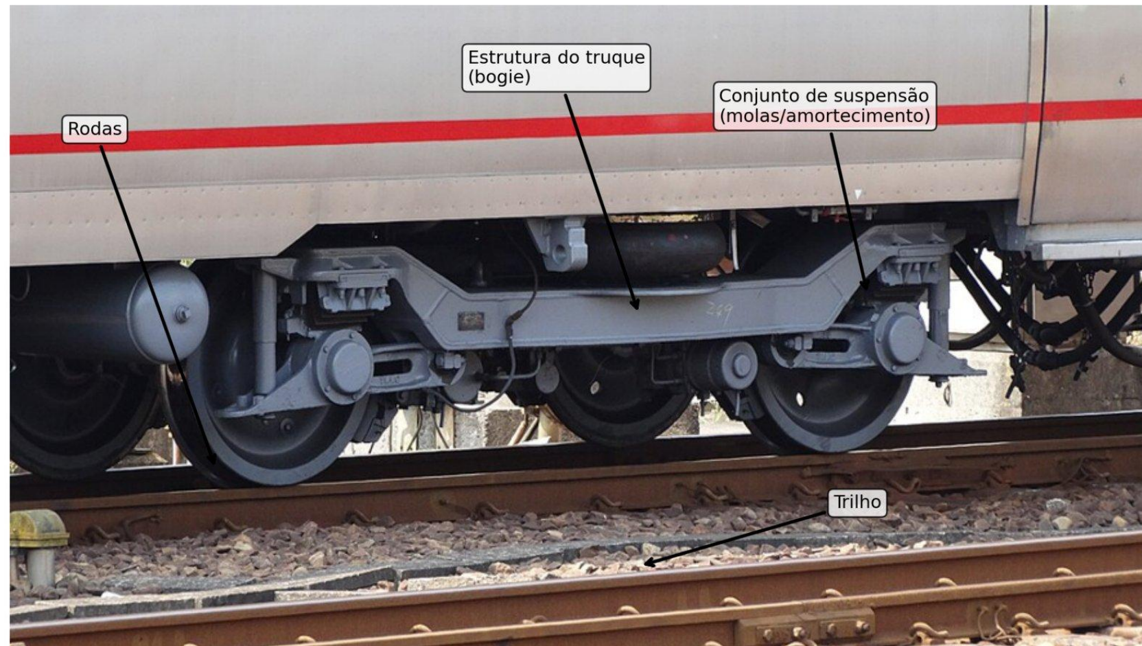
Truque ferroviário: molas, amortecedores, rodeiro
