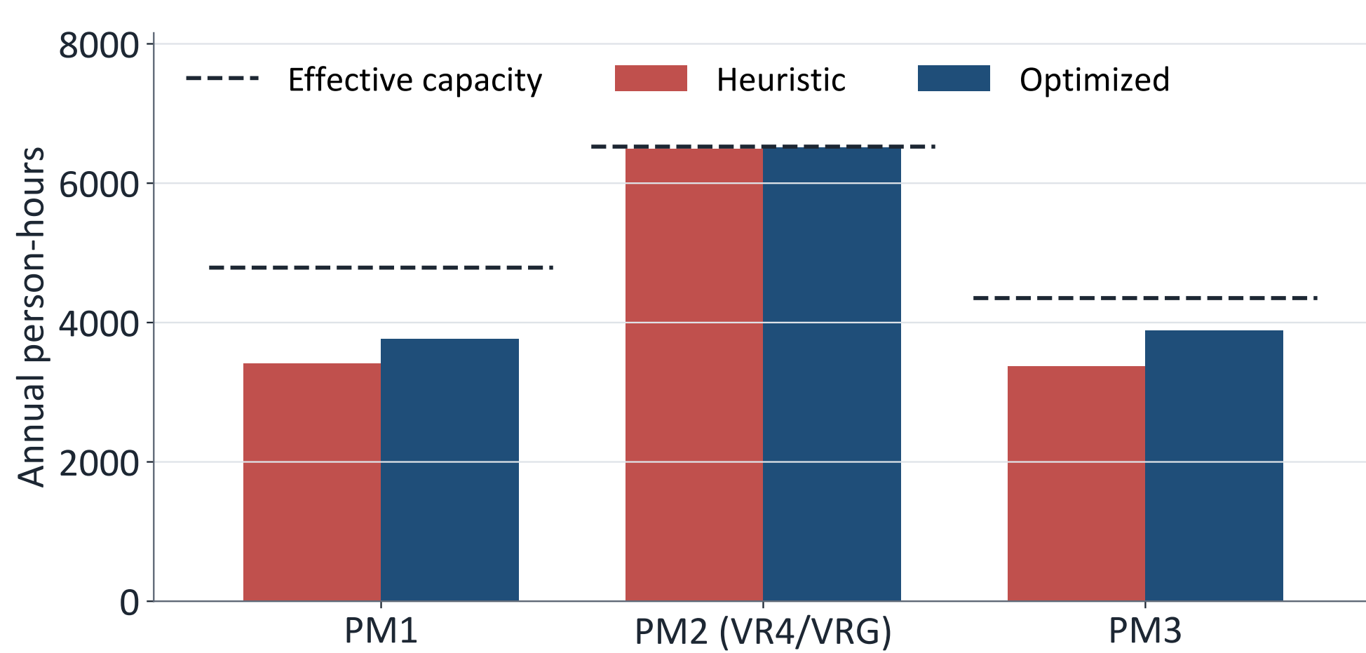
(b) HH anual por posto. A heurística ocupa o PM2 (único posto de revisão pesada) com 119 vagões leves; o ótimo envia só 34 e faz 75 VR4 em vez de 40. Heuristic fills PM2 (only heavy-scope post) with 119 light wagons; optimum sends 34 and completes 75 VR4 instead of 40.
