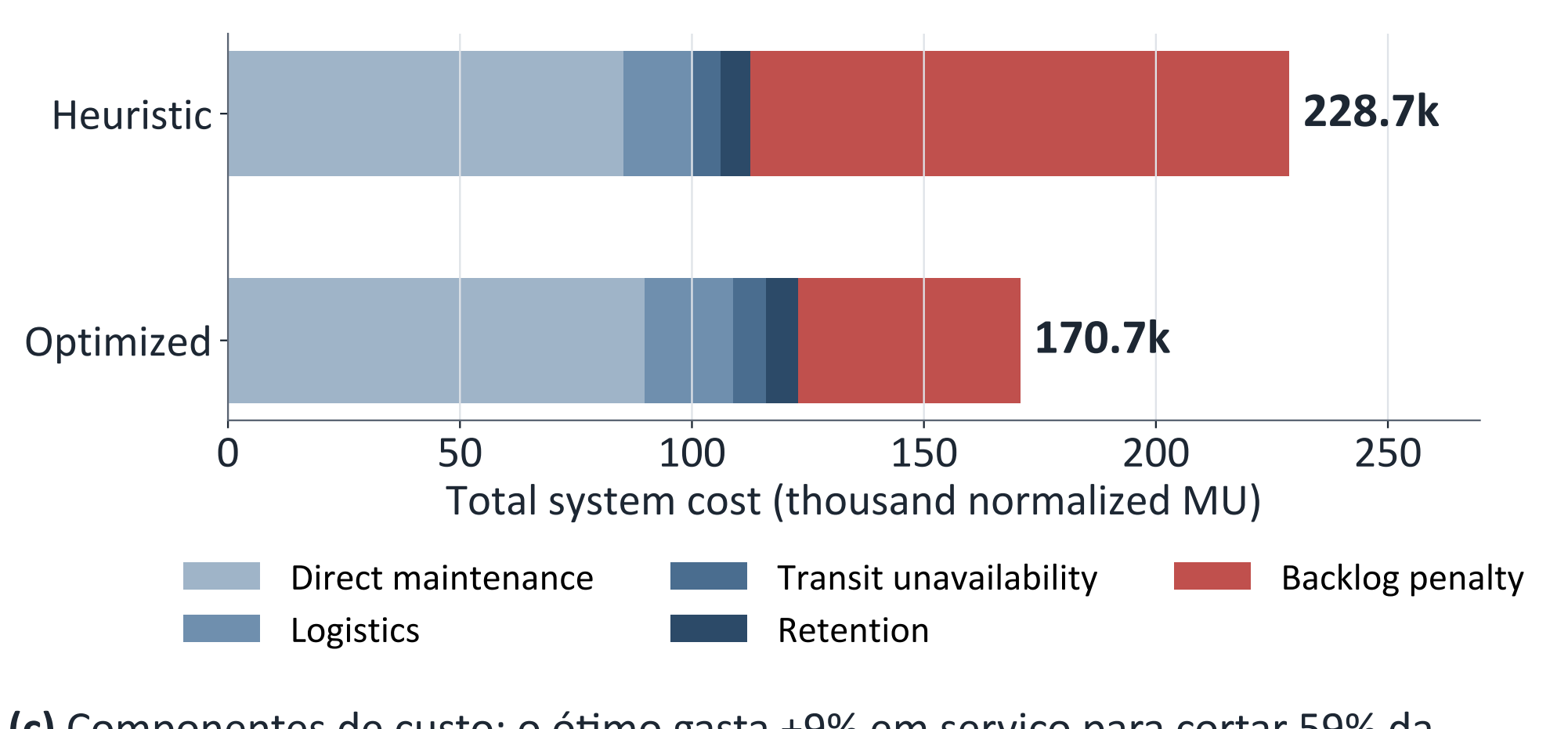
(c) Componentes de custo: o ótimo gasta +9% em serviço para cortar 59% da penalidade de backlog. Cost components: +9% service cost buys −59% backlog penalty.
