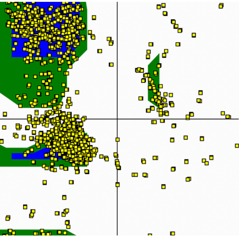
DIAGRAMA DE RAMACHANDRAN
